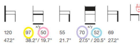
Dimensions globales
